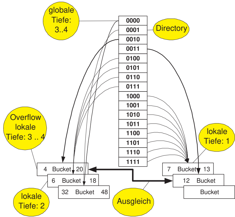
Abbildung 8.15: Erweiterbare Hash-Struktur nach der Verdoppelung des Directories
