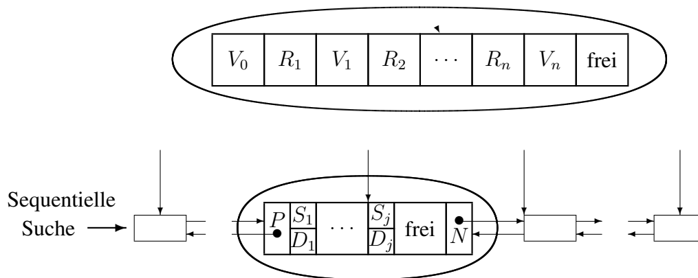
Abbildung 7.16: Schematischer Aufbau eines B + -Baums
