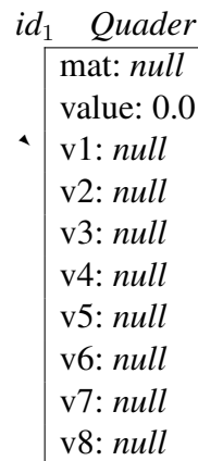
Abbildung 1.4: Die strukturelle Modellierung eines Quader-Objekts
