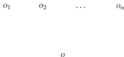
Abbildung 1.15: Gemeinsames Unterobjekt
